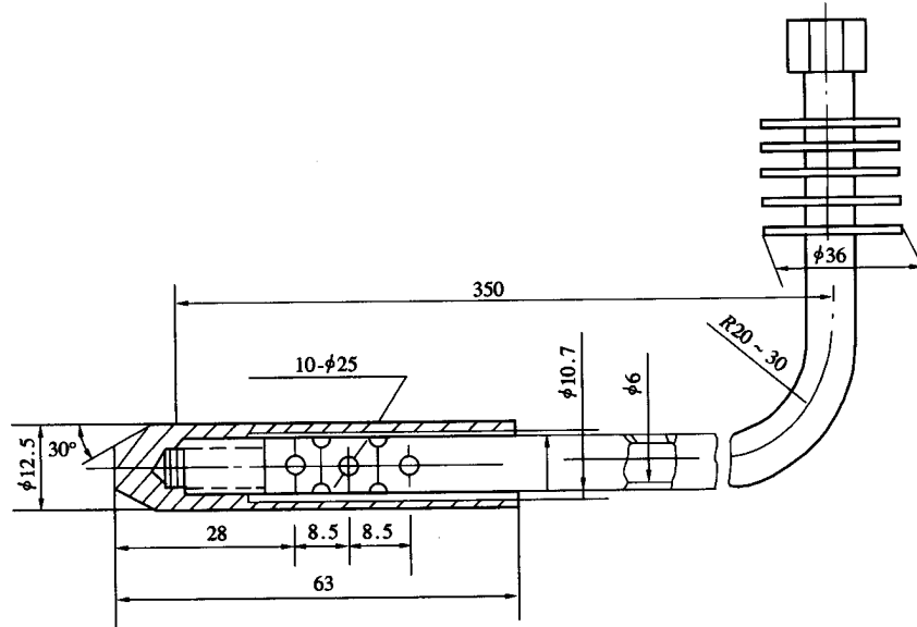
图1 取样探头
